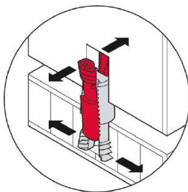
2. Empuje los componentes del panel a la vez, ambos componentes del conector se expanden simultáneamente en el agujero de perforación.
